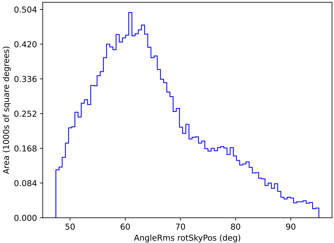
extra_ss_neo3_v3.4_10yrs WFD z band: AngleRms rotSkyPos
