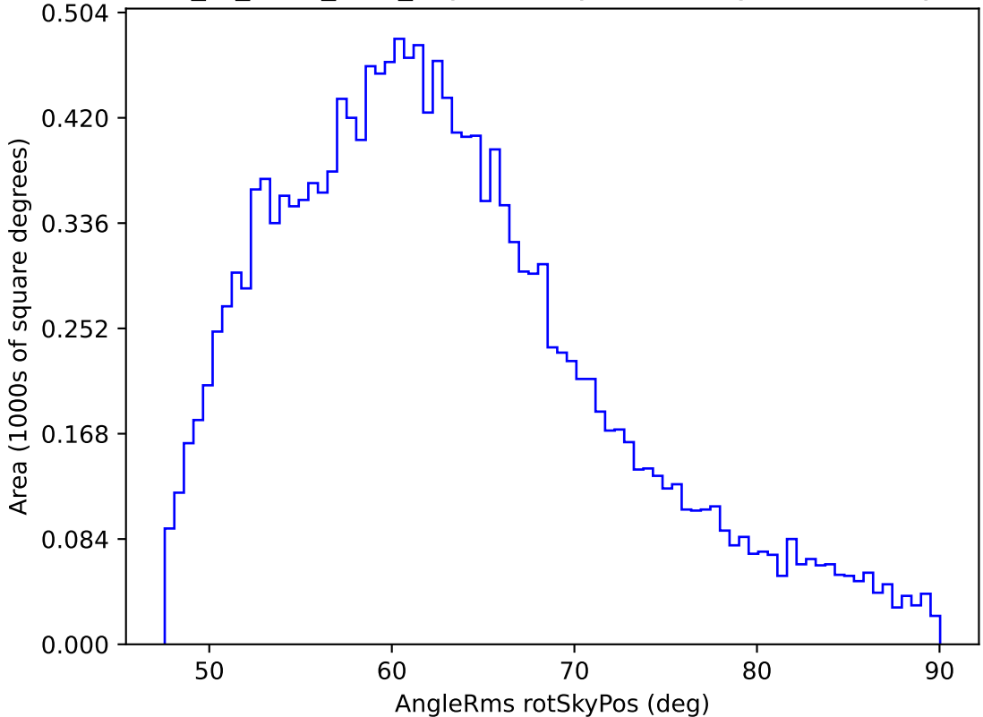
extra_ss_neo3_v3.4_10yrs WFD y band: AngleRms rotSkyPos
