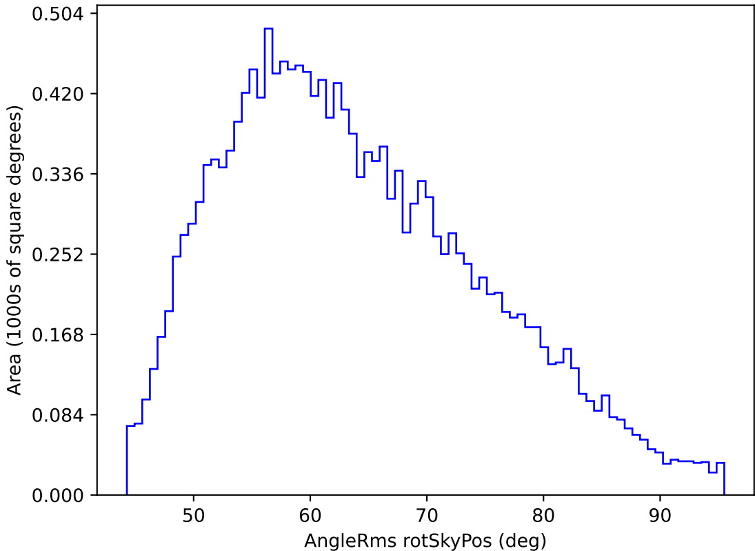
extra_ss_neo3_v3.4_10yrs WFD u band: AngleRms rotSkyPos
