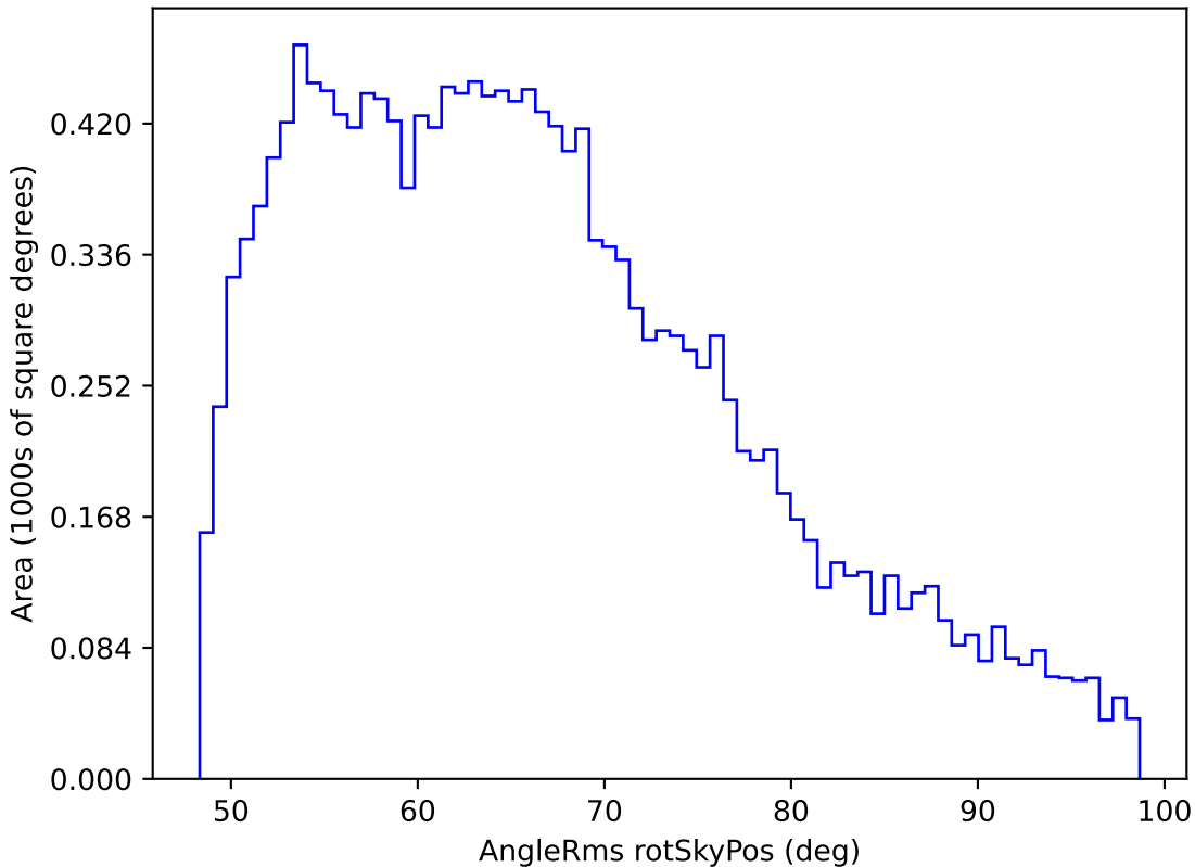
extra_ss_neo3_v3.4_10yrs WFD r band: AngleRms rotSkyPos
