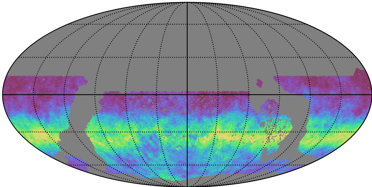
extra_ss_neo3_v3.4_10yrs WFD g band: AngleRms rotSkyPos
