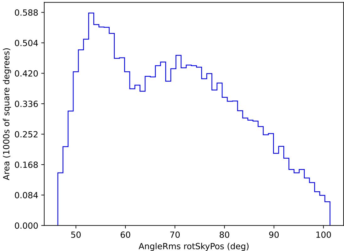
extra_ss_neo3_v3.4_10yrs WFD g band: AngleRms rotSkyPos
