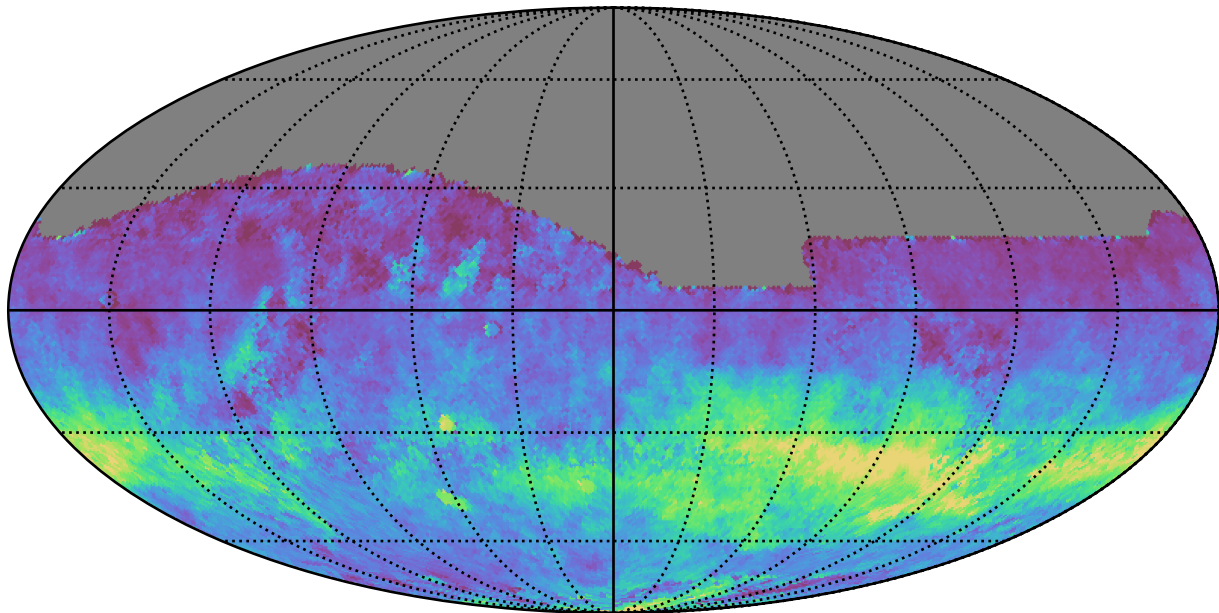
extra_ss_neo3_v3.4_10yrs All sky z band: AngleRms rotSkyPos
