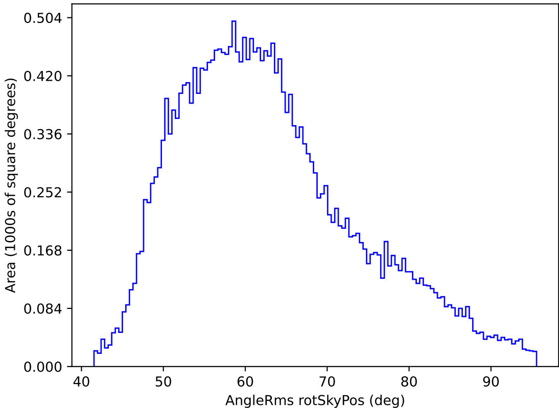
extra_ss_neo3_v3.4_10yrs All sky z band: AngleRms rotSkyPos
