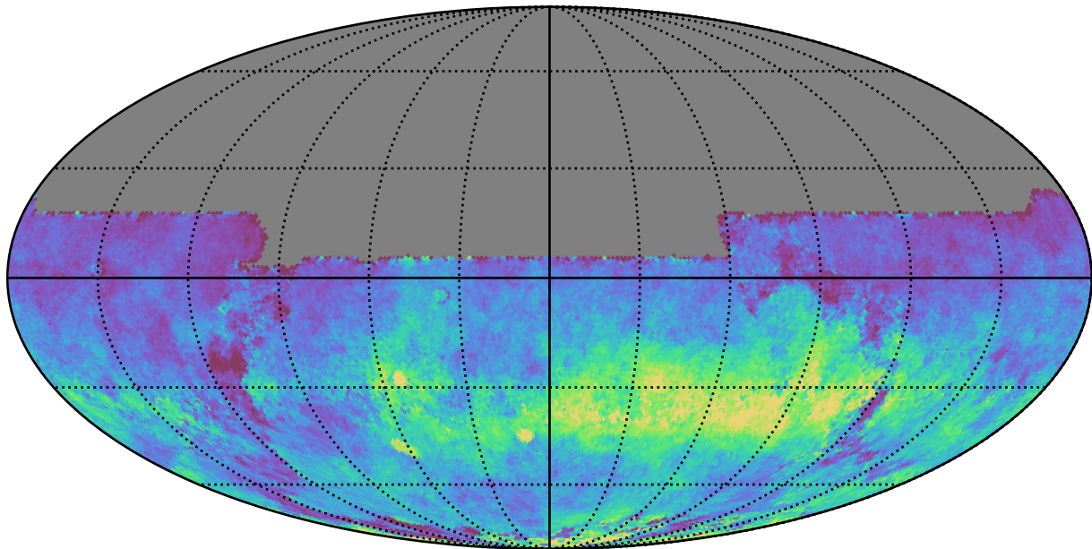
extra_ss_neo3_v3.4_10yrs All sky y band: AngleRms rotSkyPos
