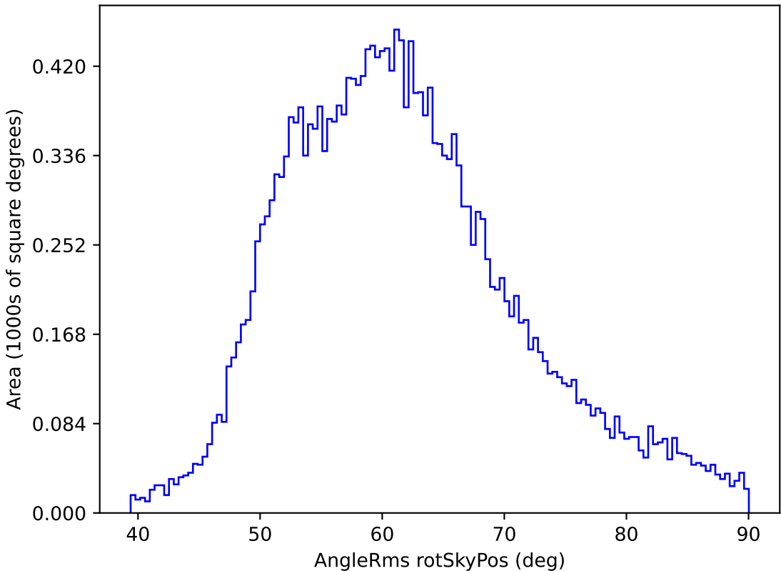
extra_ss_neo3_v3.4_10yrs All sky y band: AngleRms rotSkyPos
