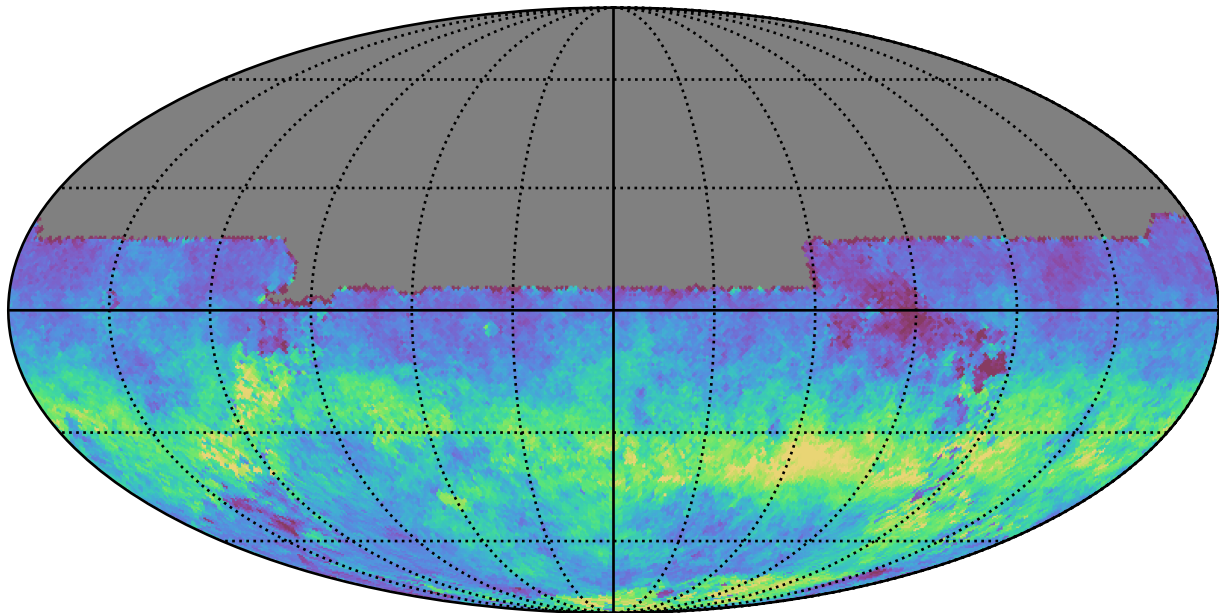
extra_ss_neo3_v3.4_10yrs All sky u band: AngleRms rotSkyPos
