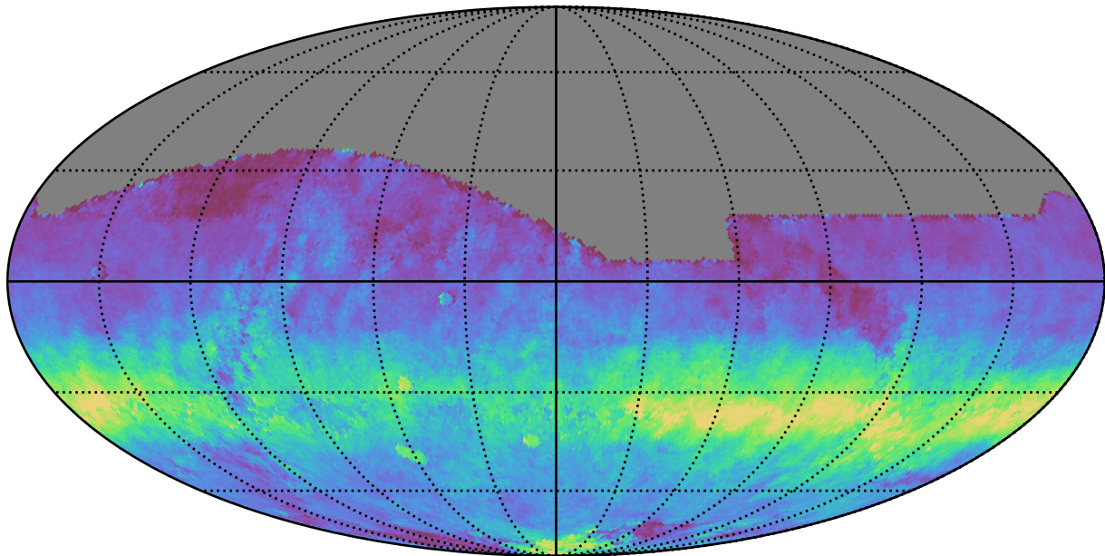
extra_ss_neo3_v3.4_10yrs All sky r band: AngleRms rotSkyPos
