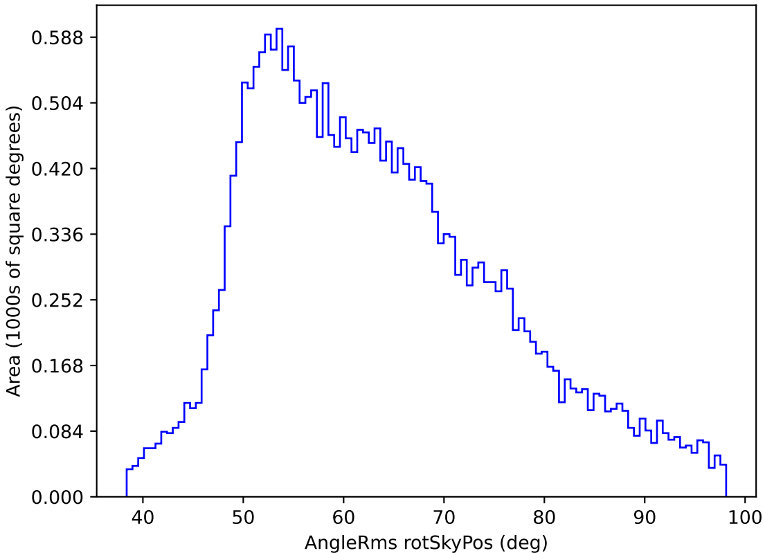
extra_ss_neo3_v3.4_10yrs All sky r band: AngleRms rotSkyPos
