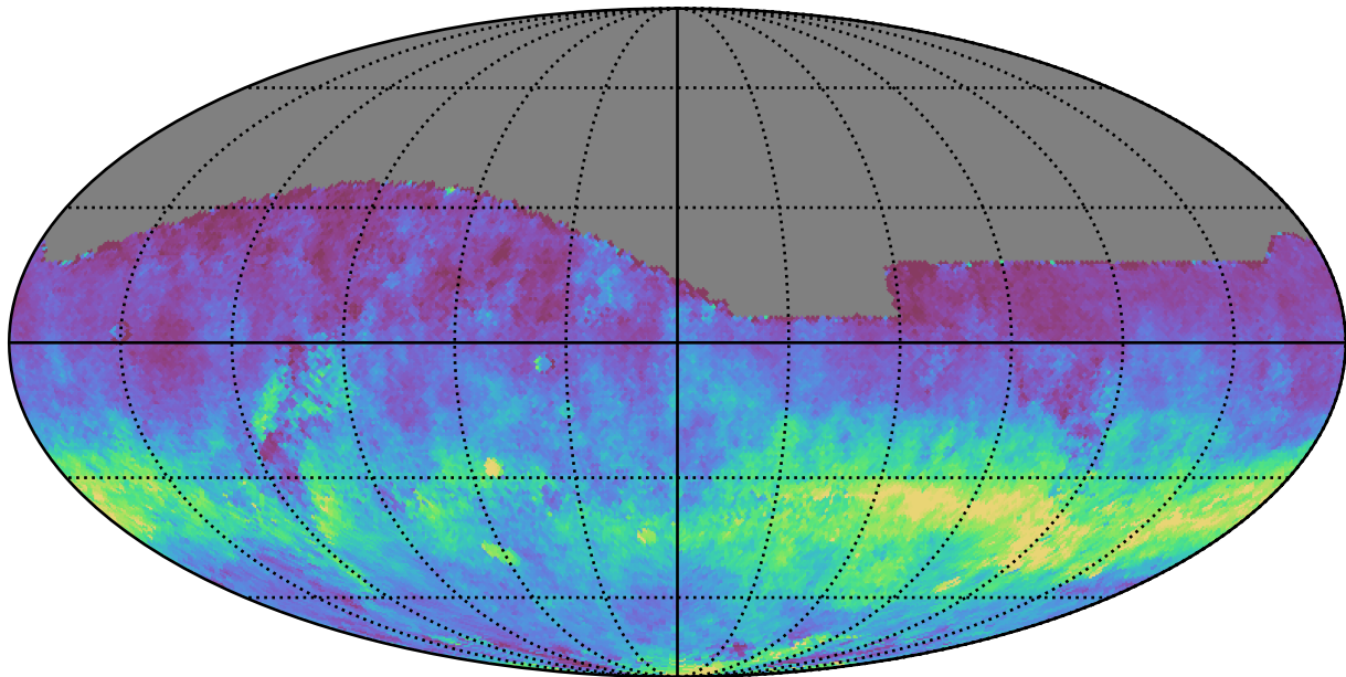
extra_ss_neo3_v3.4_10yrs All sky i band: AngleRms rotSkyPos
