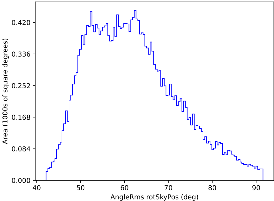
extra_ss_neo3_v3.4_10yrs All sky i band: AngleRms rotSkyPos
