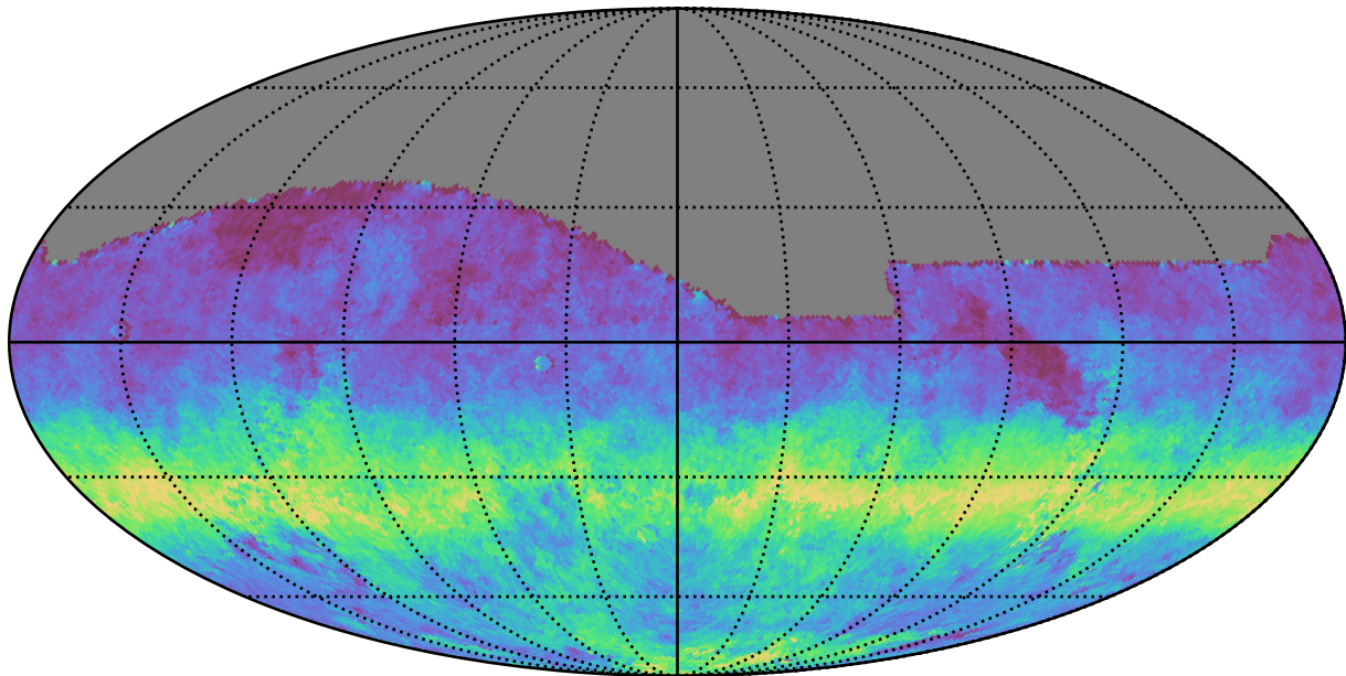
extra_ss_neo3_v3.4_10yrs All sky g band: AngleRms rotSkyPos
