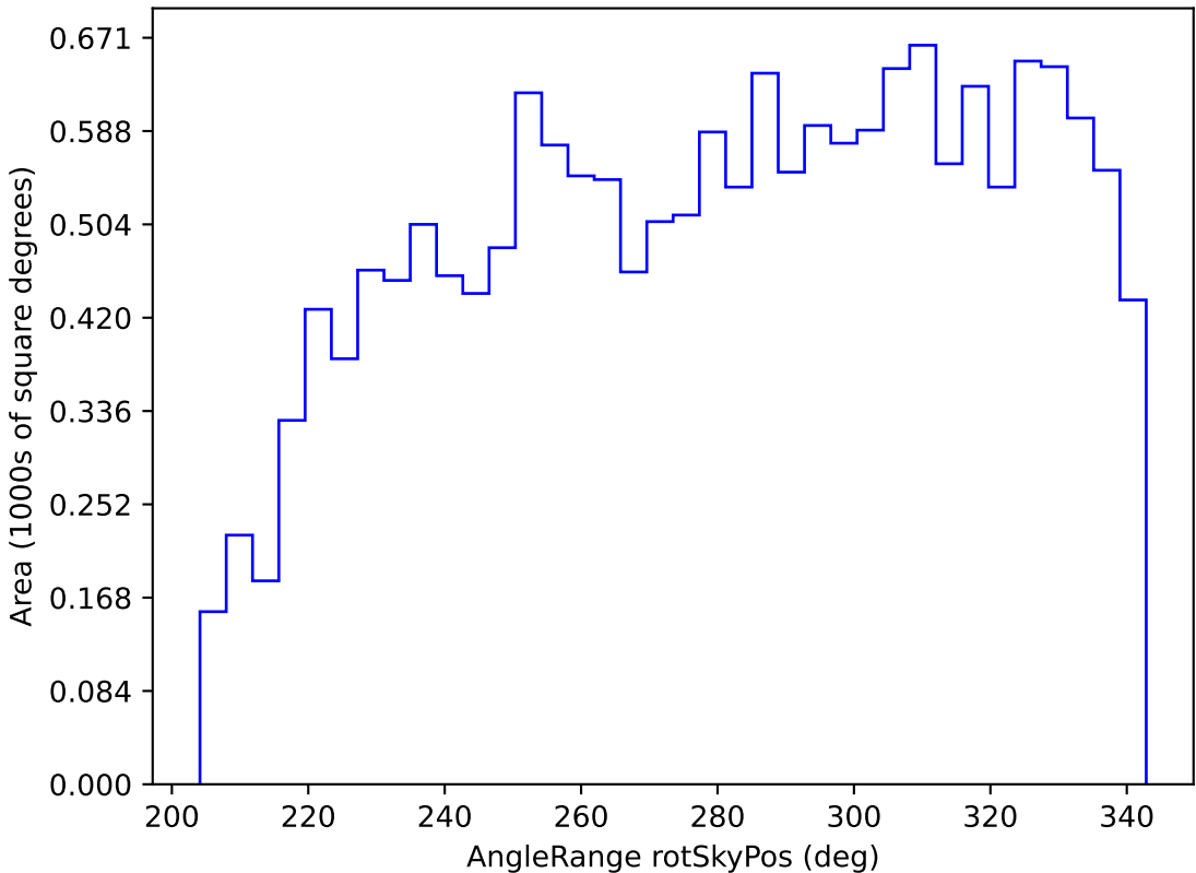
extra_ss_neo3_v3.4_10yrs WFD z band: AngleRange rotSkyPos
