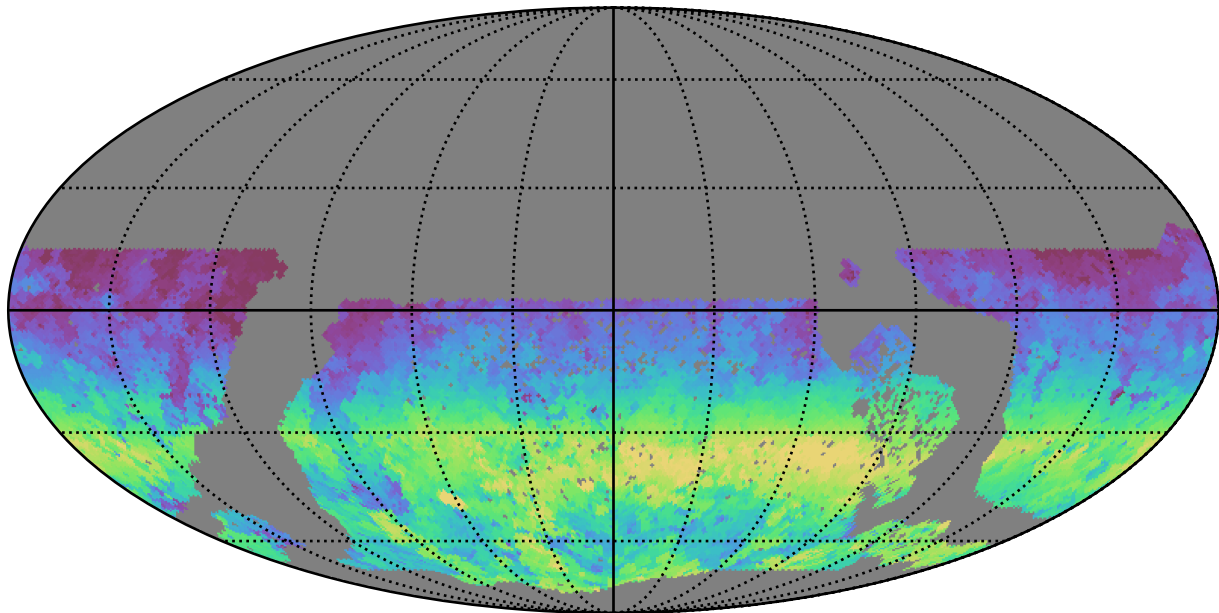
extra_ss_neo3_v3.4_10yrs WFD y band: AngleRange rotSkyPos
