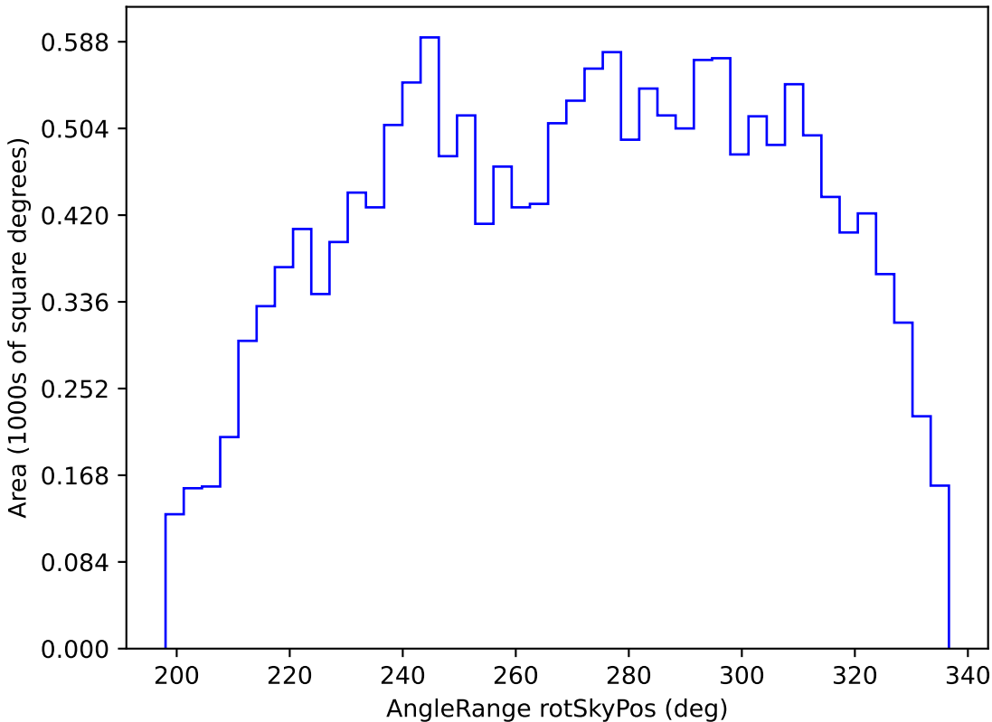
extra_ss_neo3_v3.4_10yrs WFD y band: AngleRange rotSkyPos
