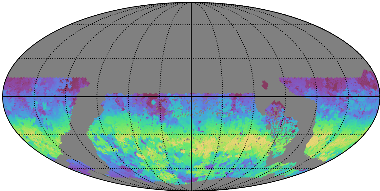
extra_ss_neo3_v3.4_10yrs WFD u band: AngleRange rotSkyPos
