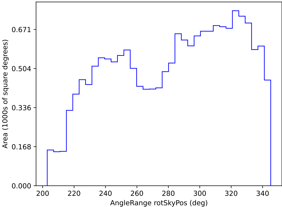
extra_ss_neo3_v3.4_10yrs WFD r band: AngleRange rotSkyPos
