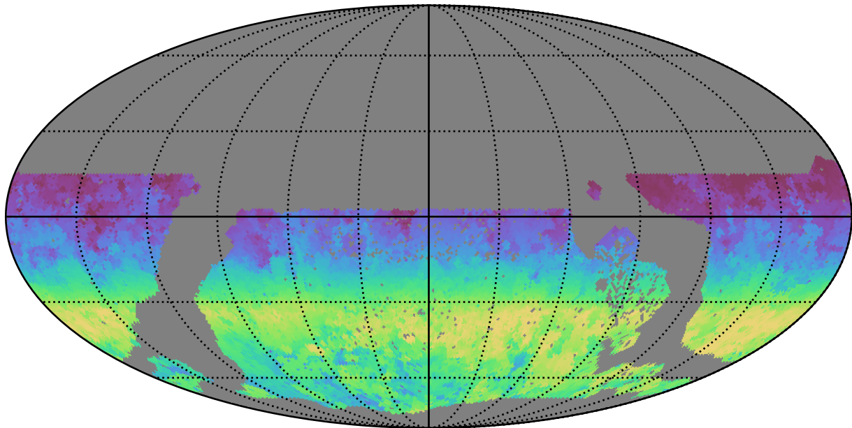
extra_ss_neo3_v3.4_10yrs WFD i band: AngleRange rotSkyPos
