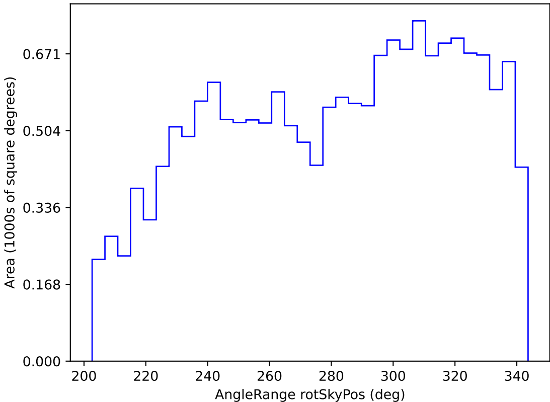
extra_ss_neo3_v3.4_10yrs WFD i band: AngleRange rotSkyPos
