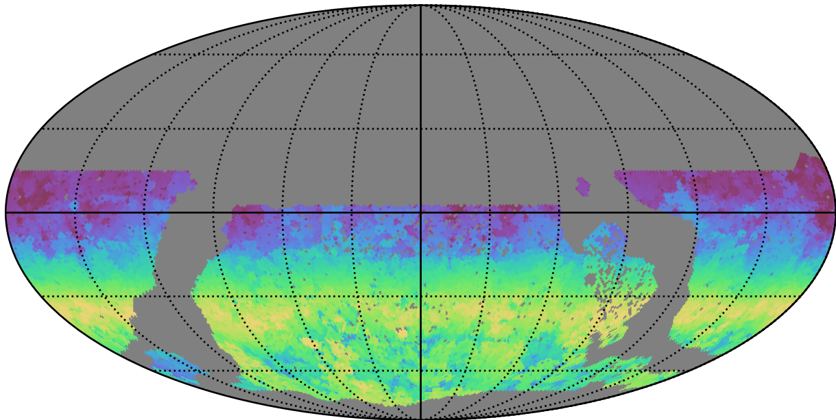
extra_ss_neo3_v3.4_10yrs WFD g band: AngleRange rotSkyPos
