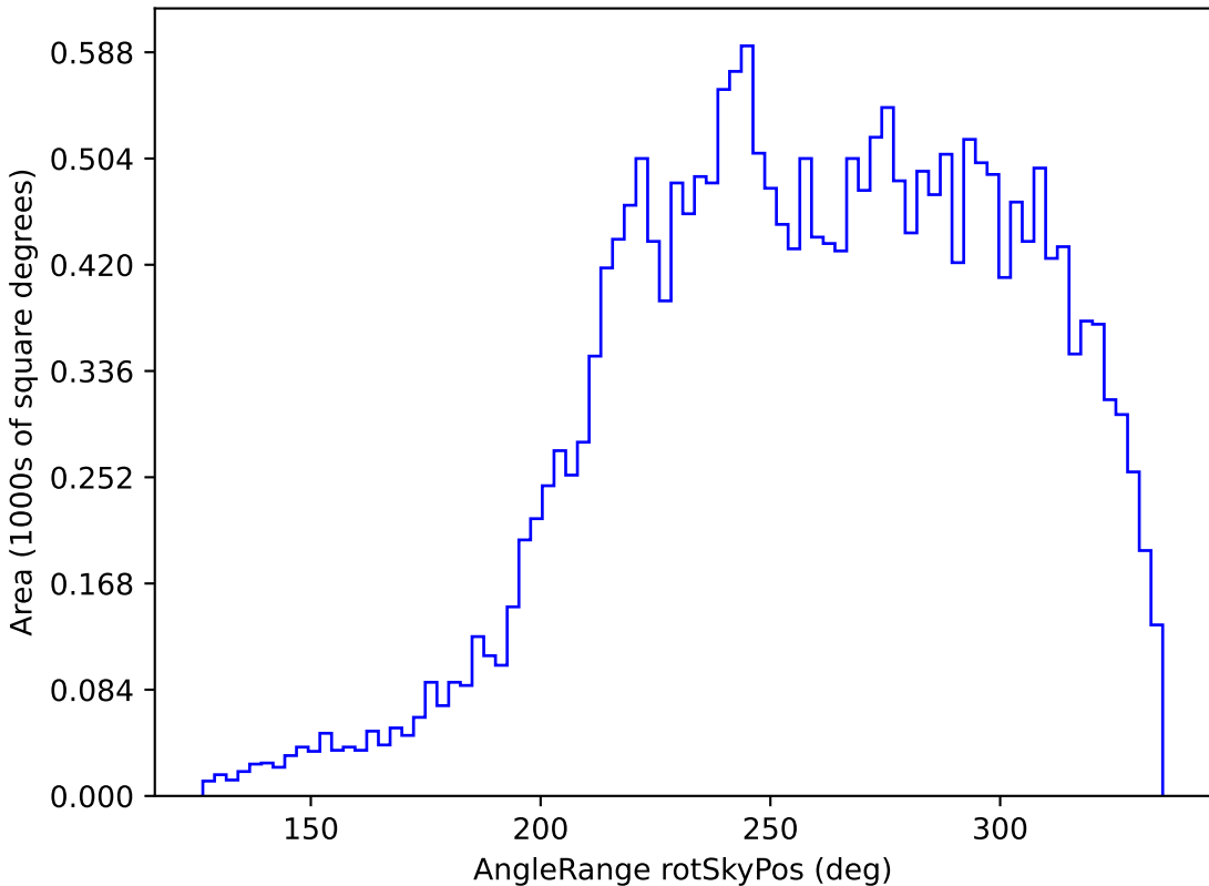
extra_ss_neo3_v3.4_10yrs All sky y band: AngleRange rotSkyPos
