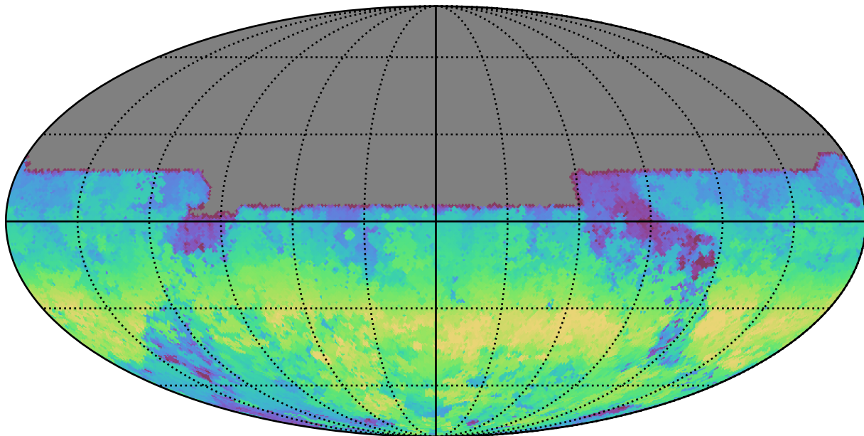
extra_ss_neo3_v3.4_10yrs All sky u band: AngleRange rotSkyPos
