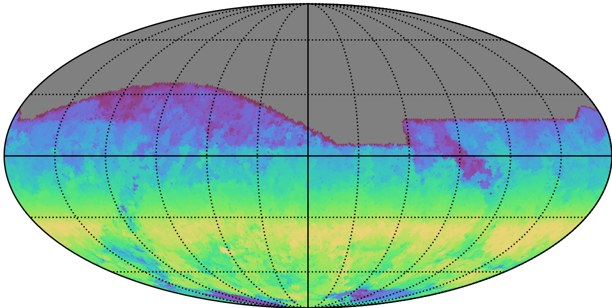
extra_ss_neo3_v3.4_10yrs All sky r band: AngleRange rotSkyPos
