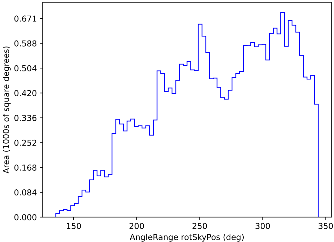
extra_ss_neo3_v3.4_10yrs All sky r band: AngleRange rotSkyPos
