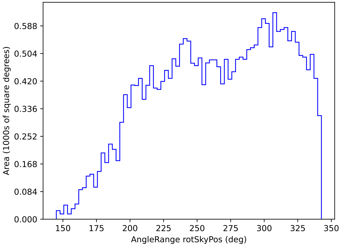
extra_ss_neo3_v3.4_10yrs All sky i band: AngleRange rotSkyPos
