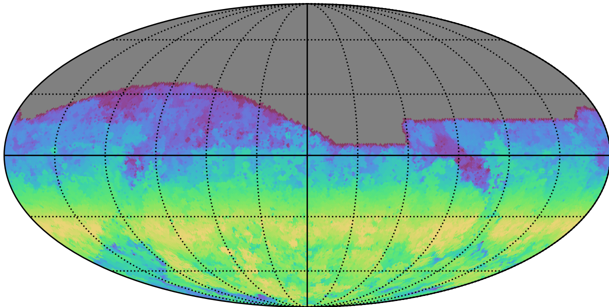
extra_ss_neo3_v3.4_10yrs All sky g band: AngleRange rotSkyPos
