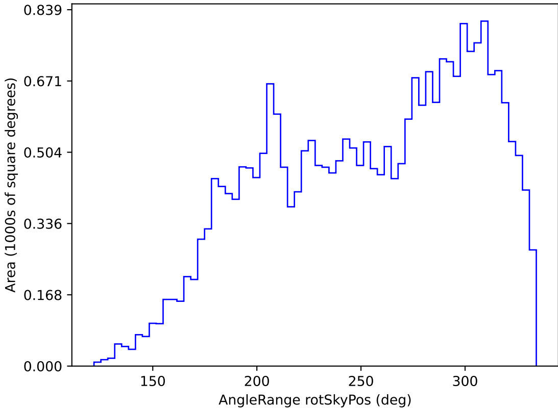
extra_ss_neo3_v3.4_10yrs All sky g band: AngleRange rotSkyPos
