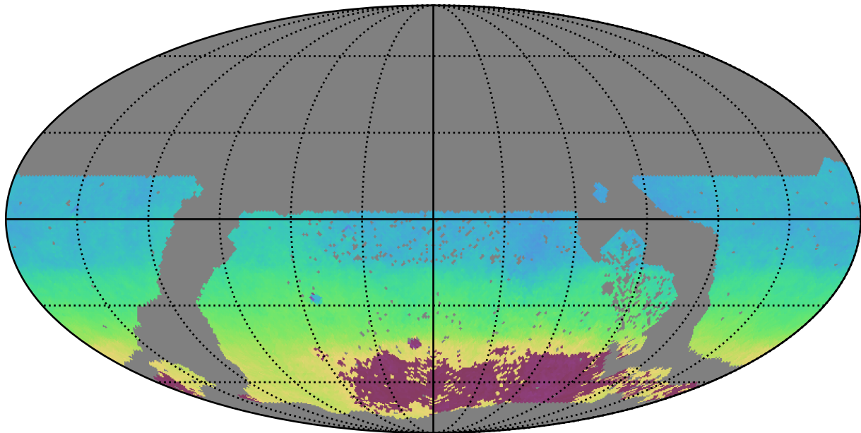
extra_ss_neo3_v3.4_10yrs WFD y band: AngleMean rotSkyPos
