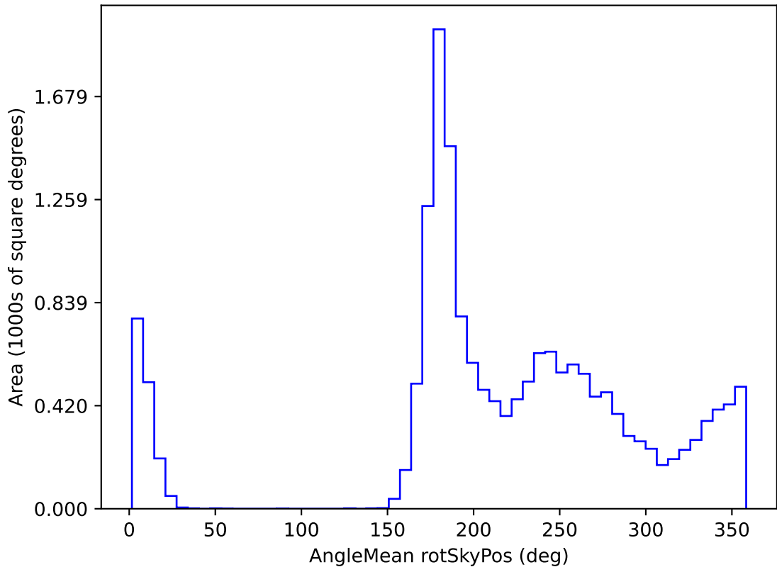
extra_ss_neo3_v3.4_10yrs WFD y band: AngleMean rotSkyPos
