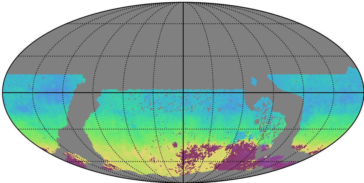
extra_ss_neo3_v3.4_10yrs WFD u band: AngleMean rotSkyPos
