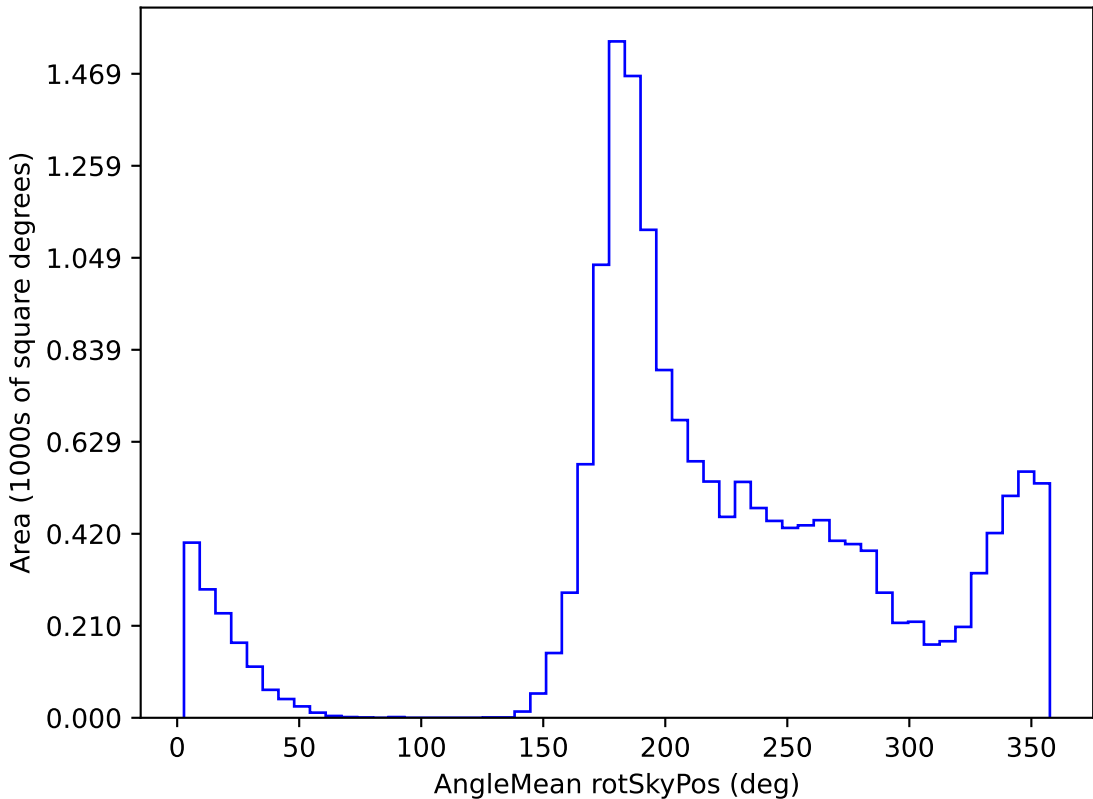
extra_ss_neo3_v3.4_10yrs WFD u band: AngleMean rotSkyPos
