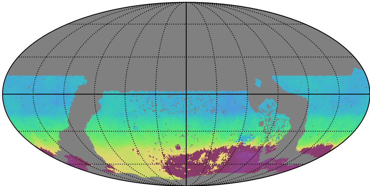
extra_ss_neo3_v3.4_10yrs WFD r band: AngleMean rotSkyPos
