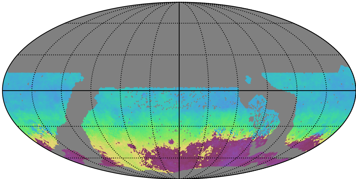
extra_ss_neo3_v3.4_10yrs WFD g band: AngleMean rotSkyPos
