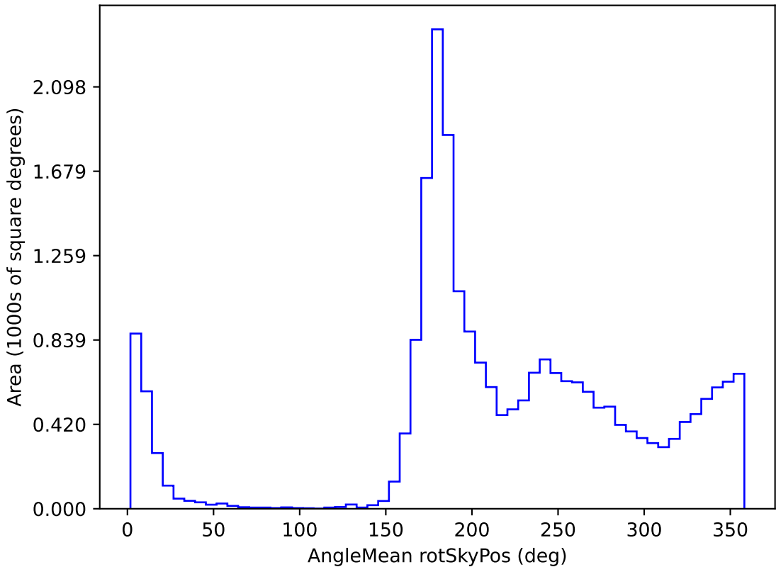
extra_ss_neo3_v3.4_10yrs All sky y band: AngleMean rotSkyPos
