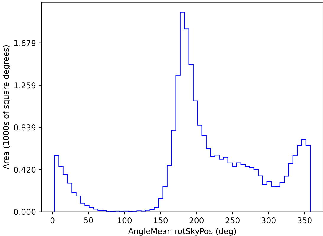
extra_ss_neo3_v3.4_10yrs All sky u band: AngleMean rotSkyPos
