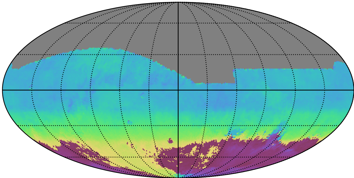
extra_ss_neo3_v3.4_10yrs All sky r band: AngleMean rotSkyPos
