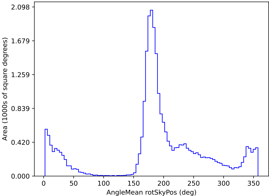
extra_ss_neo3_v3.4_10yrs All sky r band: AngleMean rotSkyPos
