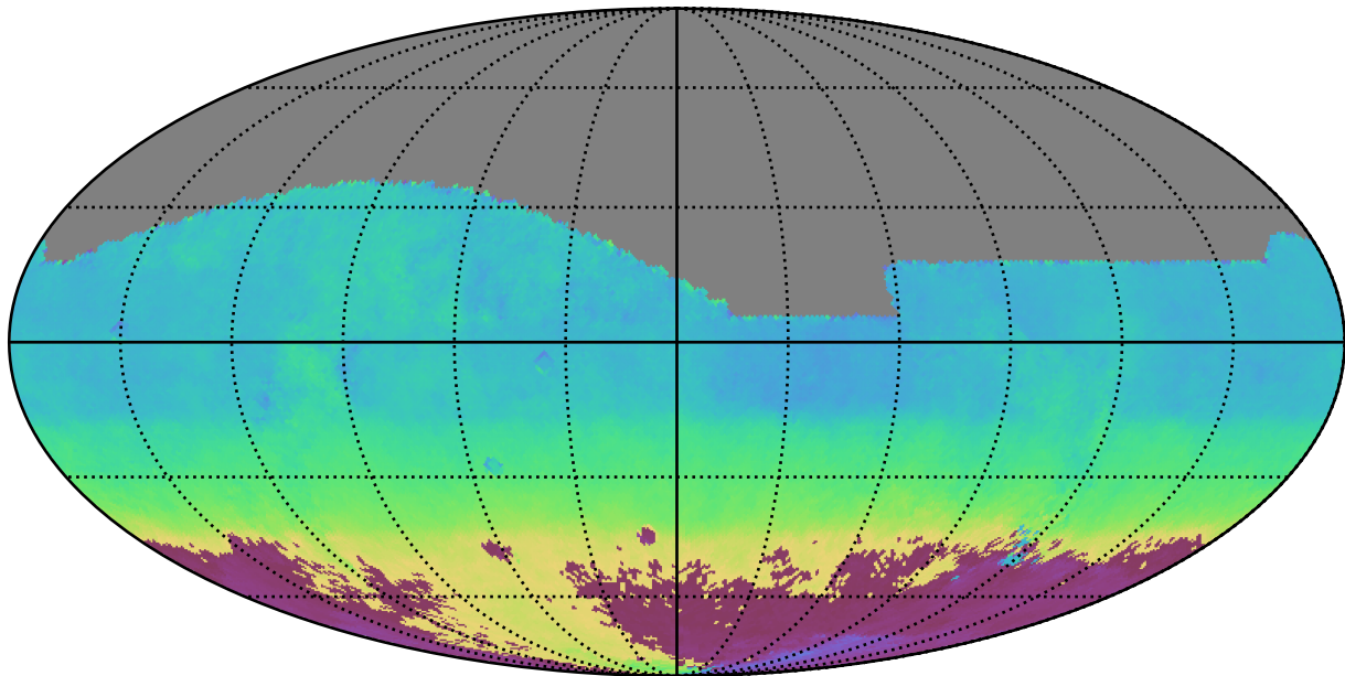
extra_ss_neo3_v3.4_10yrs All sky i band: AngleMean rotSkyPos
