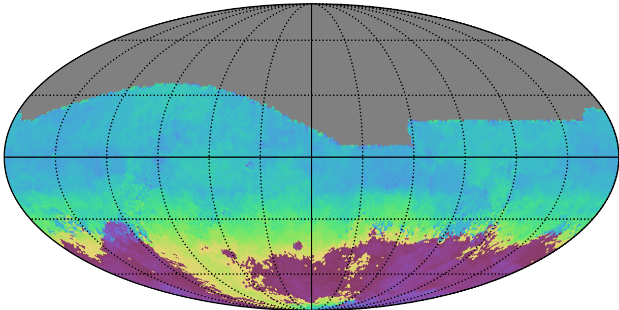
extra_ss_neo3_v3.4_10yrs All sky g band: AngleMean rotSkyPos
