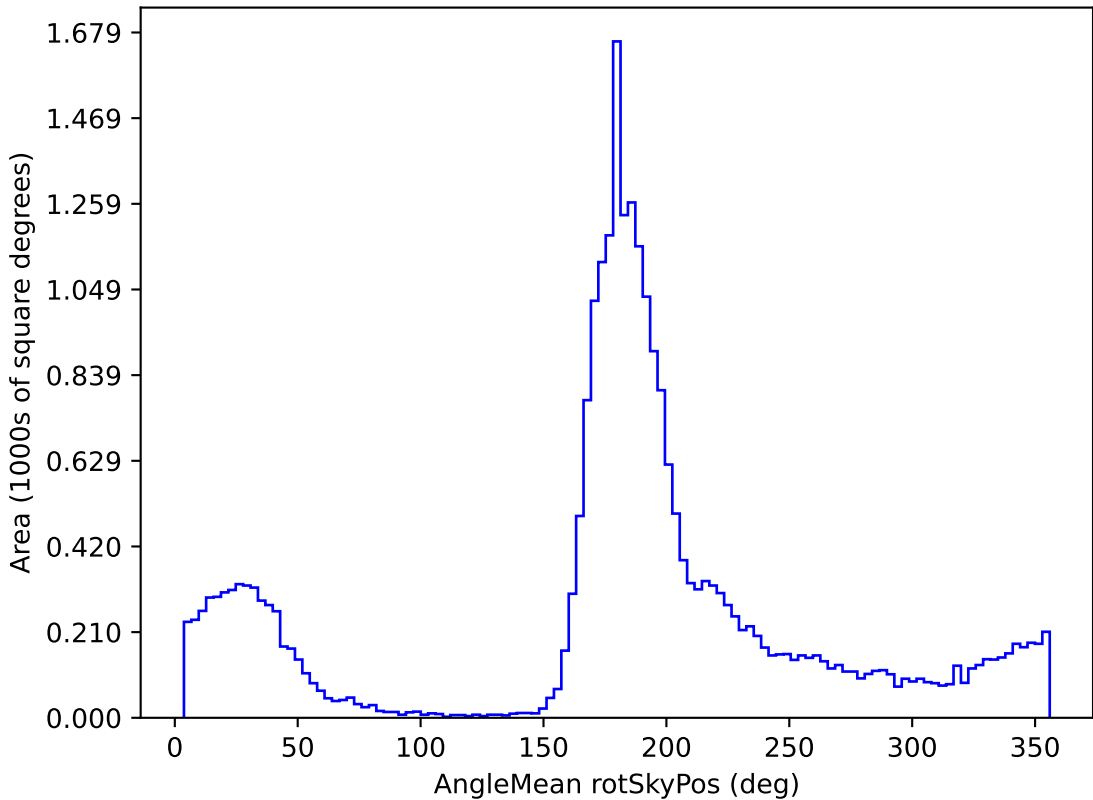
extra_ss_neo3_v3.4_10yrs All sky g band: AngleMean rotSkyPos
