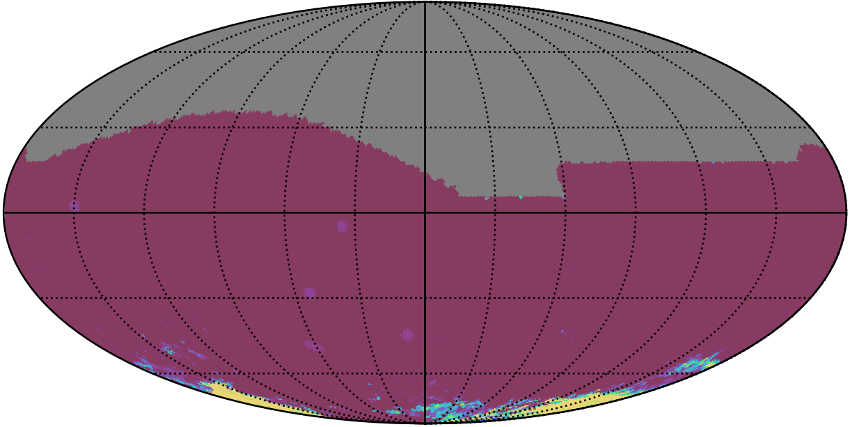
extra_ss_neo3_v3.4_10yrs All sky iz bands: 75th Percentile Intranight Timespan
