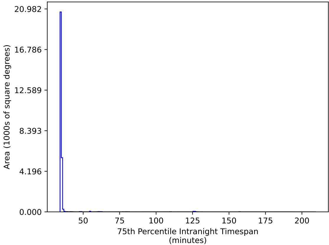
extra_ss_neo3_v3.4_10yrs All sky iz bands: 75th Percentile Intranight Timespan
