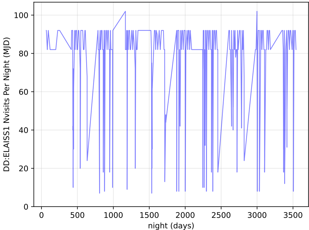
extra_ss_neo3_v3.4_10yrs all bands: DD:ELAISS1 Nvisits Per Night
