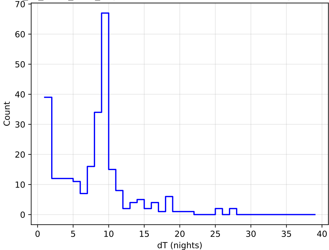
extra_ss_neo3_v3.4_10yrs all bands: DD:ELAISS1 Delta Nights Histogram
