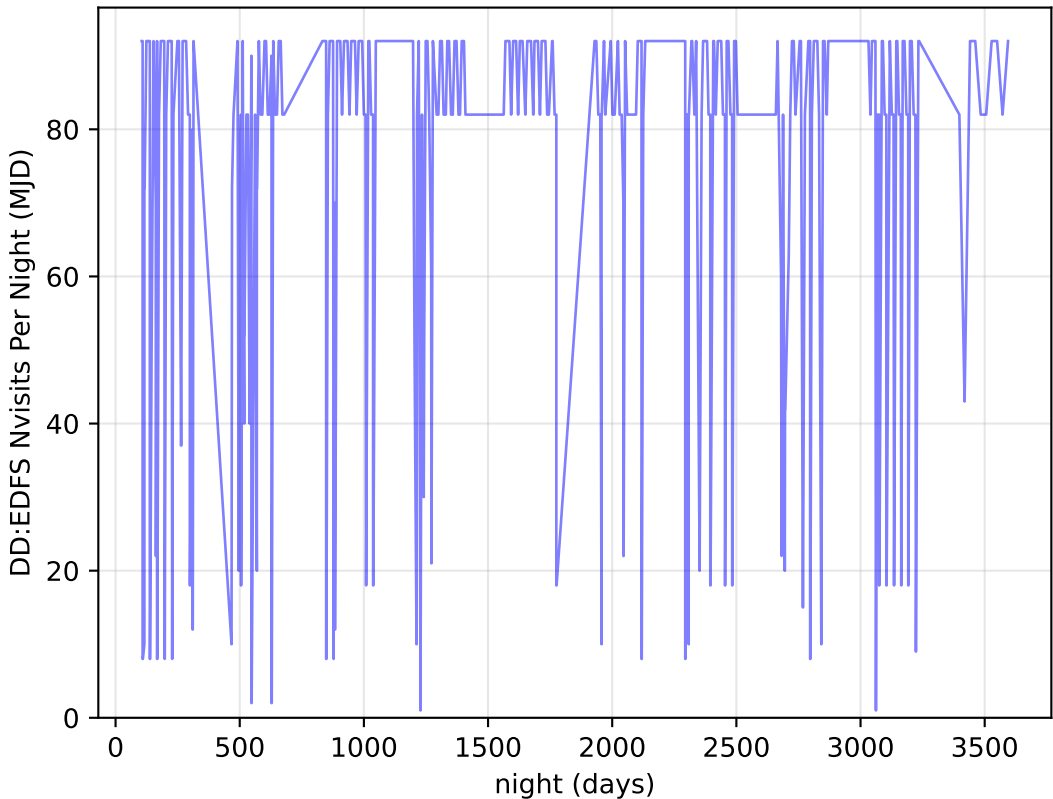
extra_ss_neo3_v3.4_10yrs all bands: DD:EDFS Nvisits Per Night
