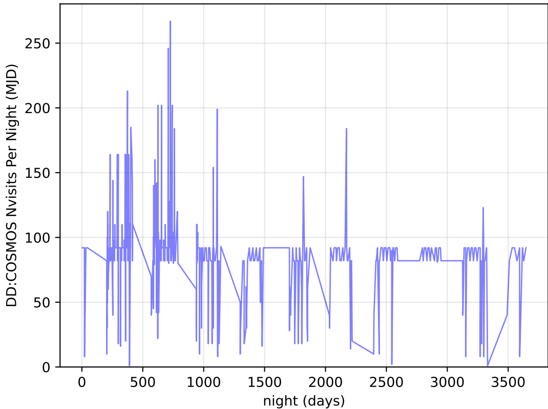
extra_ss_neo3_v3.4_10yrs all bands: DD: COSMOS Nvisits Per Night
